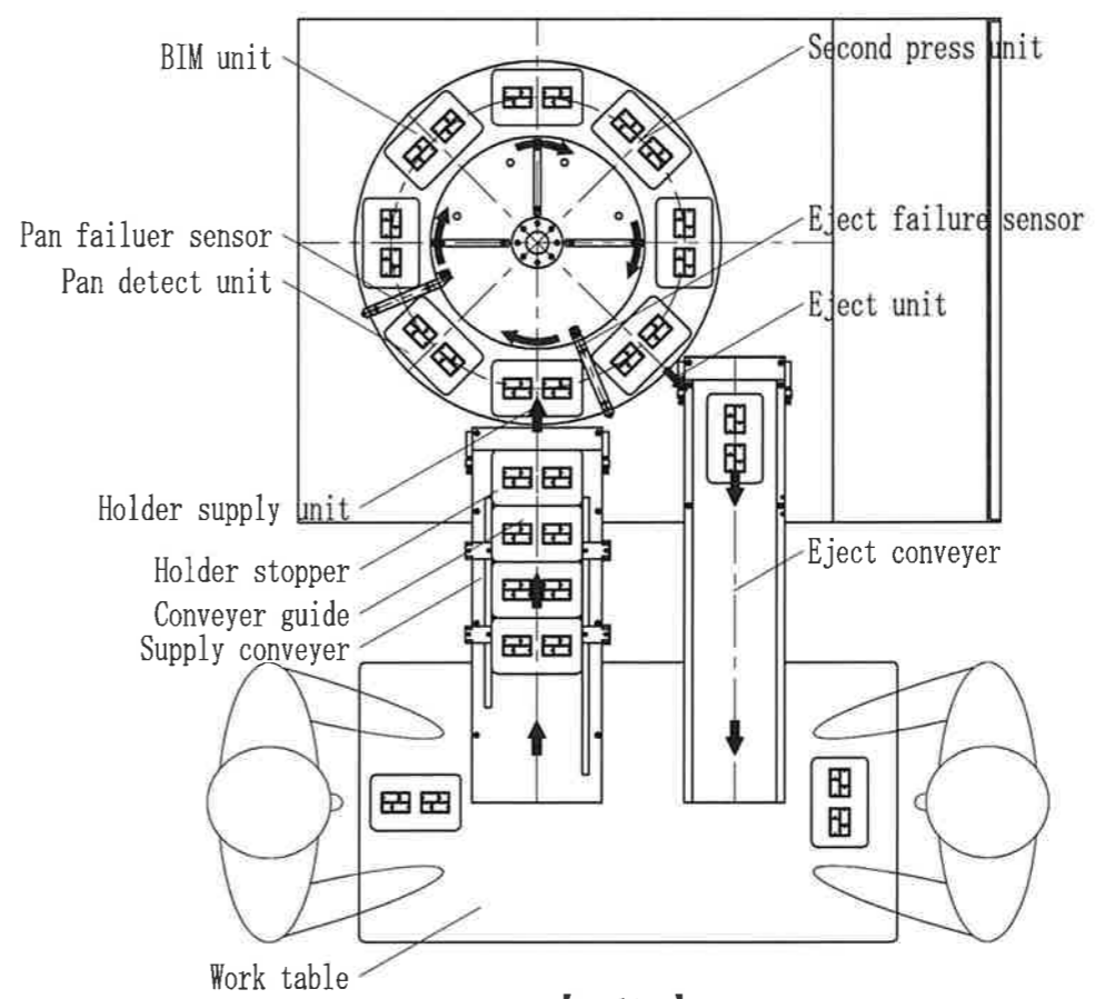
【Outline】
